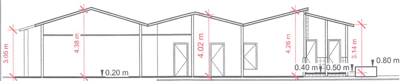
1 CORTE A 1 : 150
