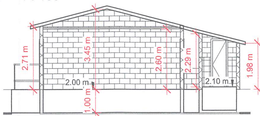
1 CORTE A 1 : 100
