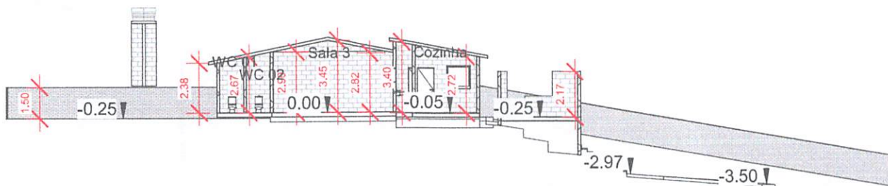
1 Corte A 1 : 250
