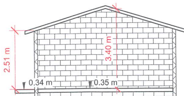
1 CORTE A 1 : 100
