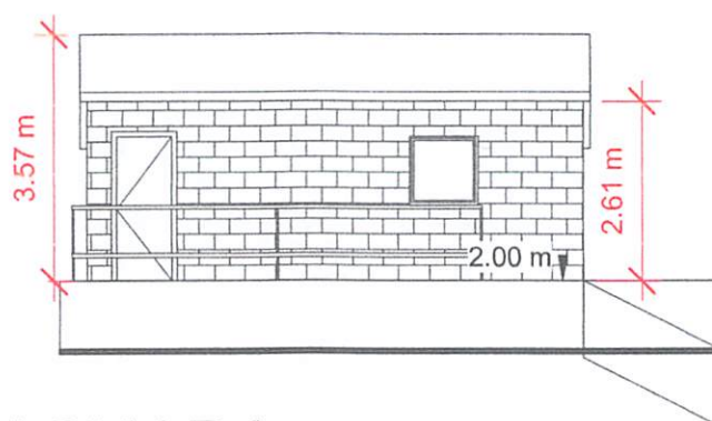
3 FACHADA 1 : 120
