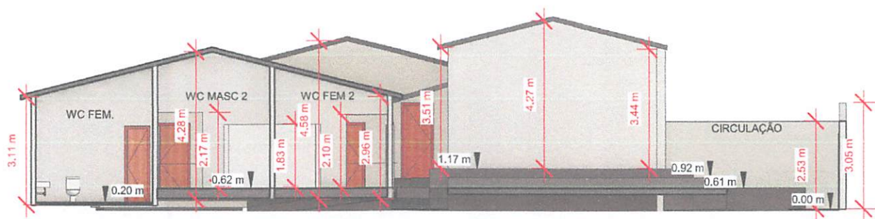
1 CORTE A 1 : 150
