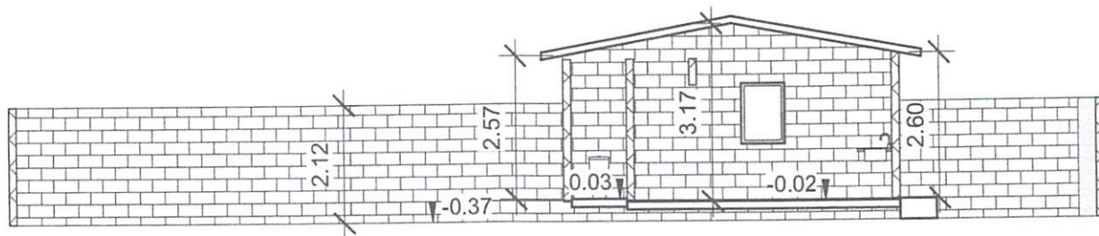
1 CORTE A 1 : 120
