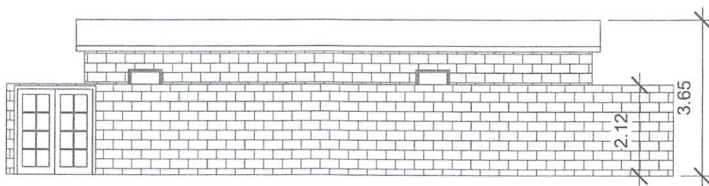
3 FACHADA 1 : 120
