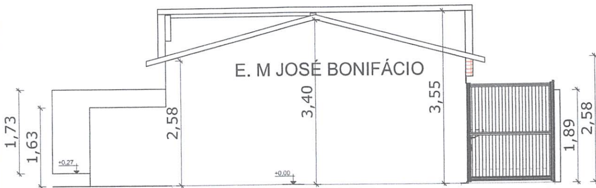
1 FACHADA FRONTAL 1 : 75
