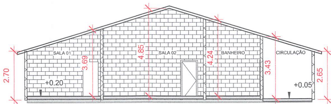
2 CORTE B 1 : 120
