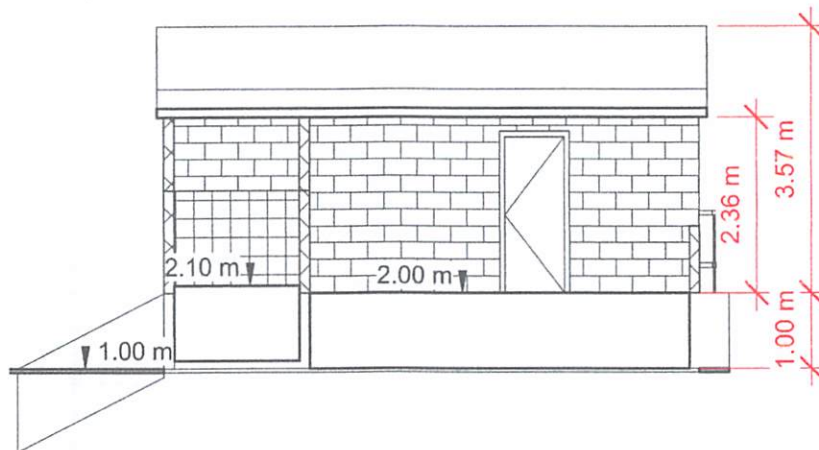
1 CORTE A 1 : 100
