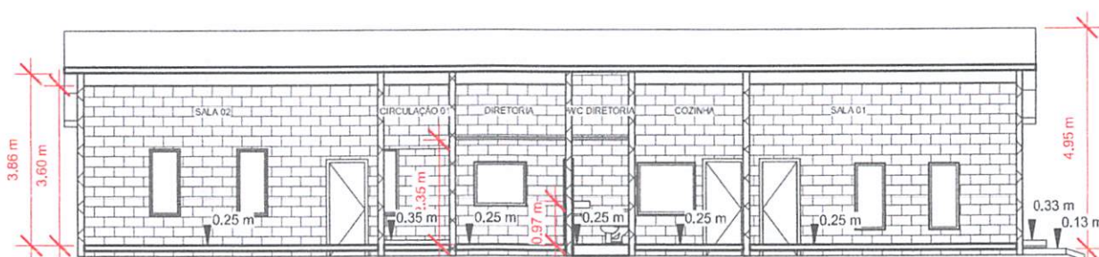
2 CORTE B 1 : 150
