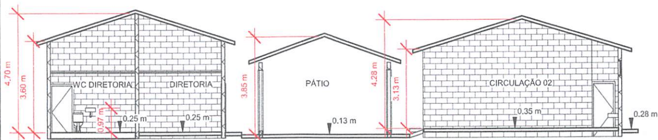
1 CORTE A 1 : 150
