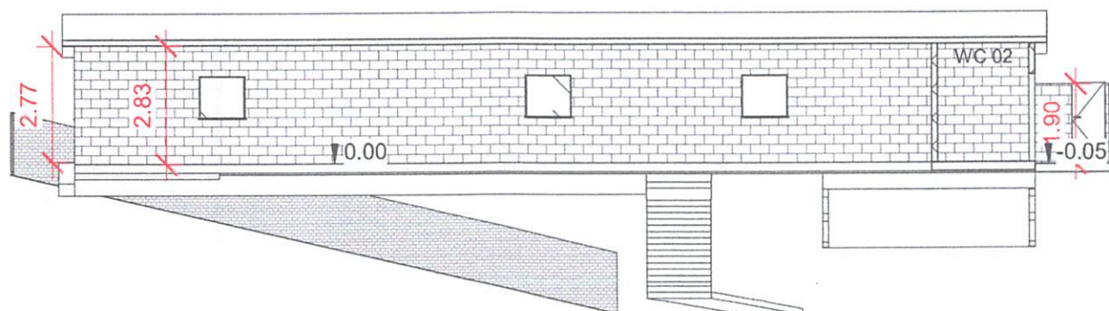
2 Corte B 1 : 160
