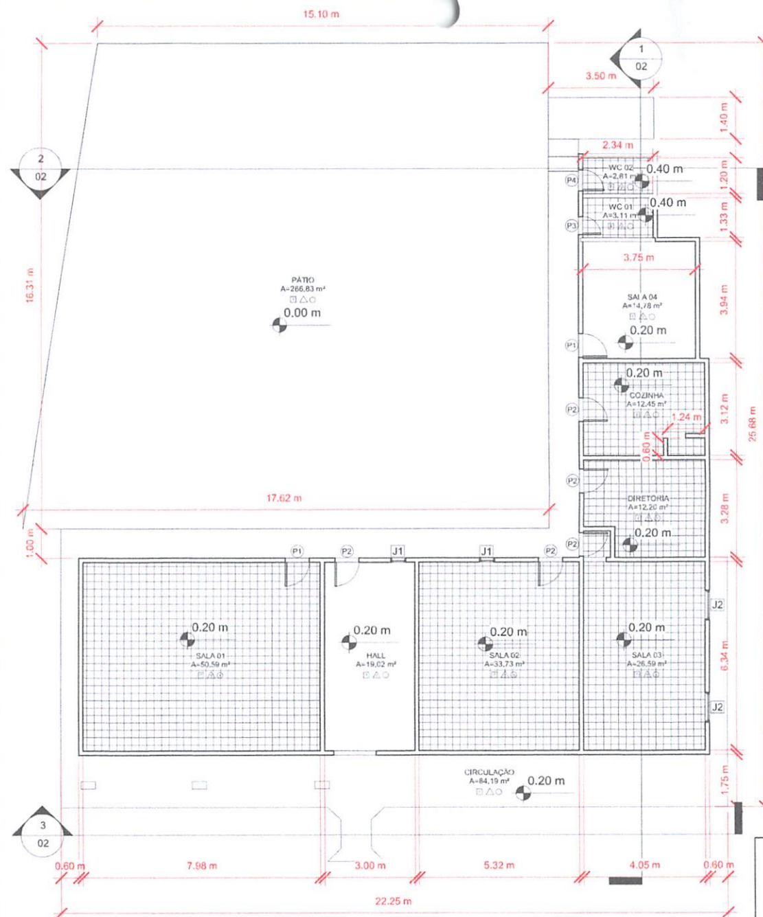
1 PLANTA BAIXA 1 : 120
