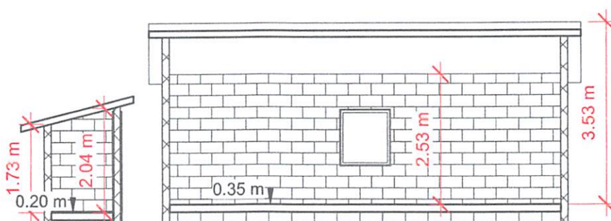
2 CORTE B 1 : 100
