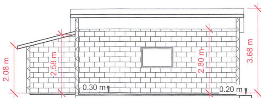
2 CORTE B 1 : 100
