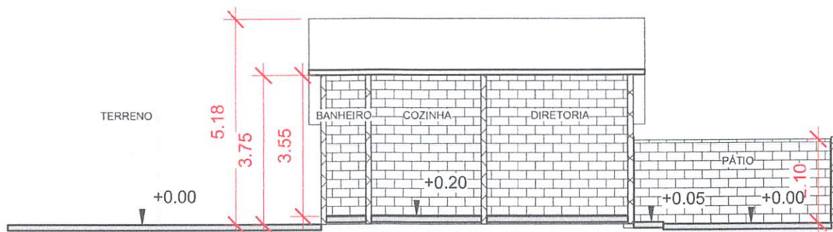
1 CORTE A 1 : 130
