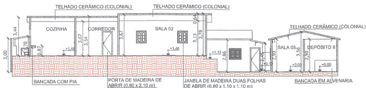
2 CORTE B 1 : 200
