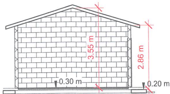
1 CORTE A 1 : 100
