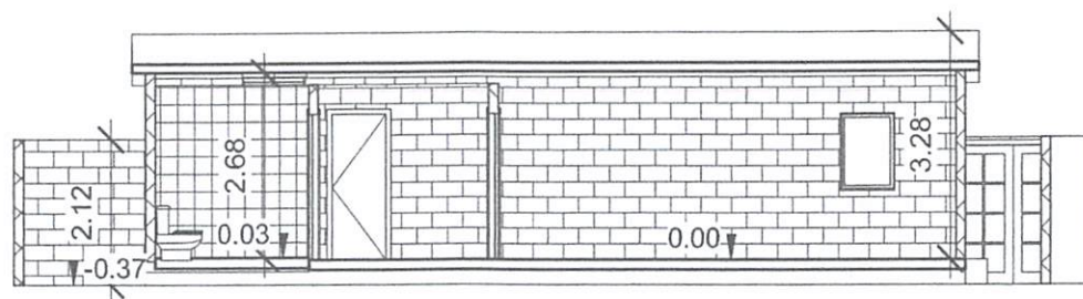
2 CORTE B 1 : 120
