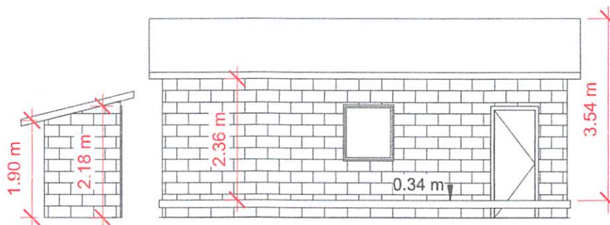
3 FACHADA 1 : 100
