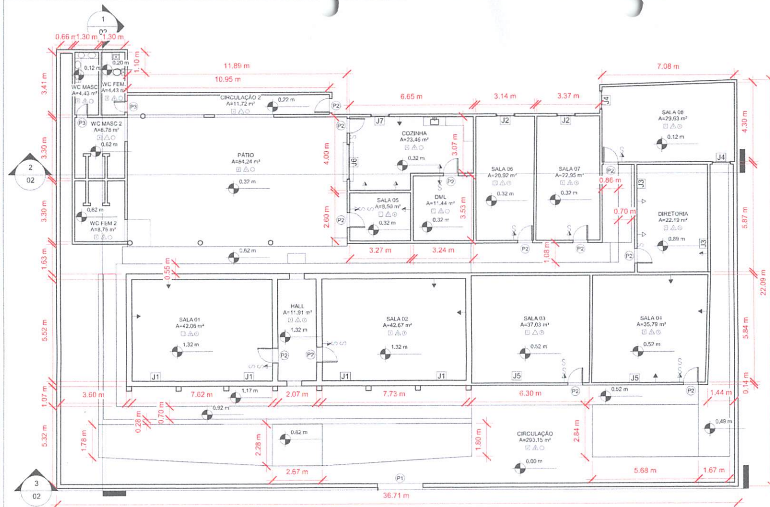
1 PLANTA BAIXA 1 : 140
