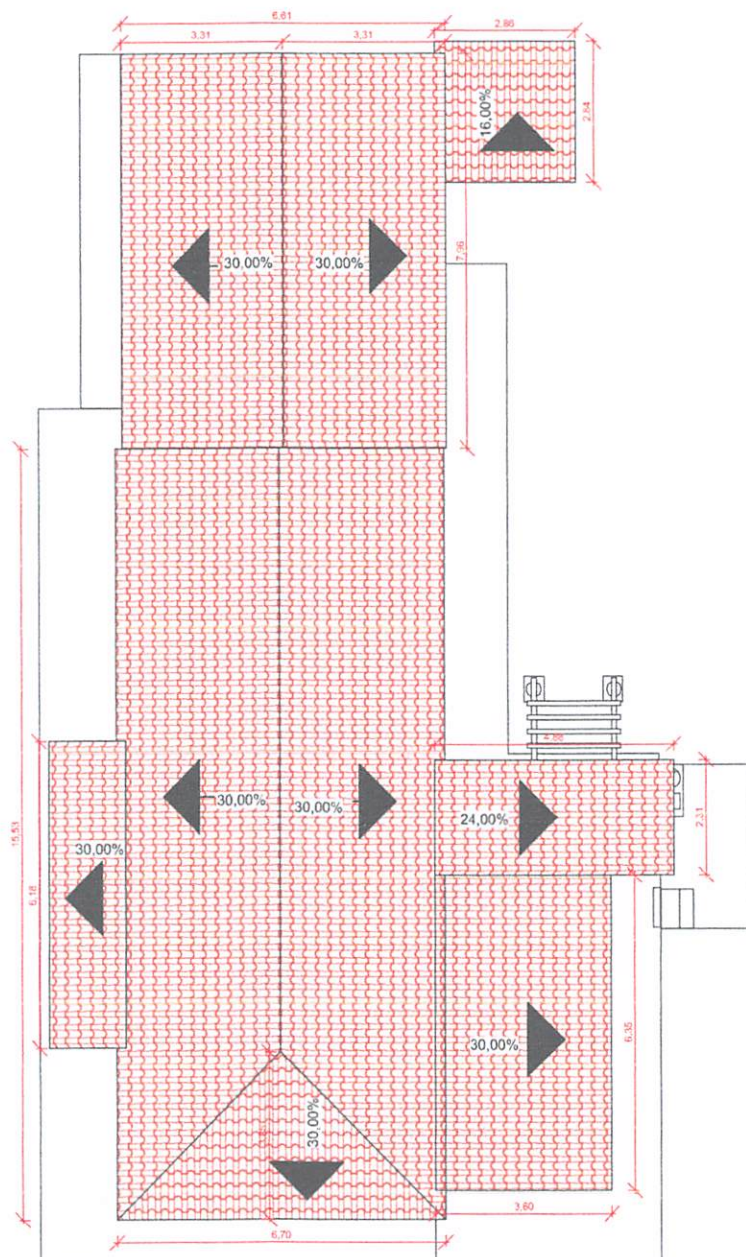
2 Cobertura 1 : 150
