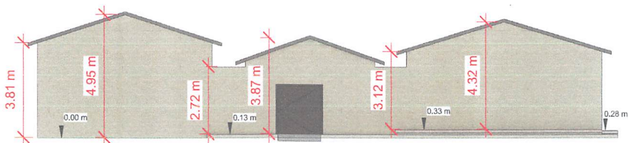
3 FACHADA 1 : 150
