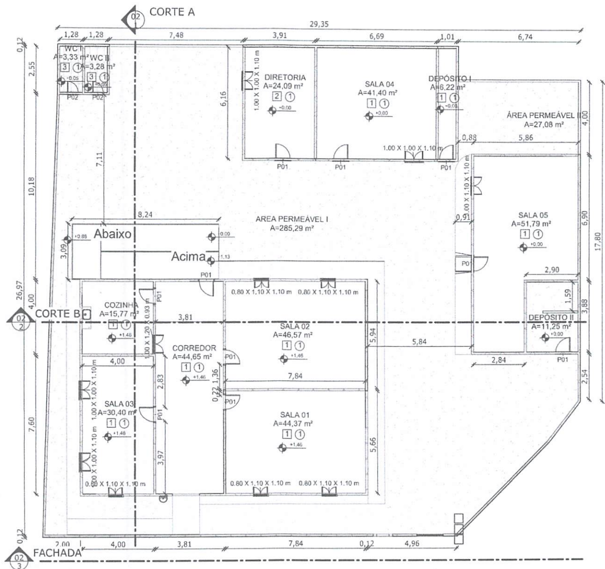
1 PLANTA BAIXA 1 : 200
