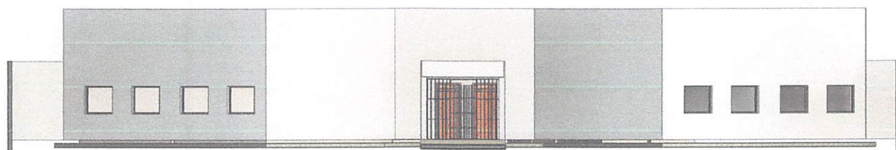
3 FACHADA 1 : 200
