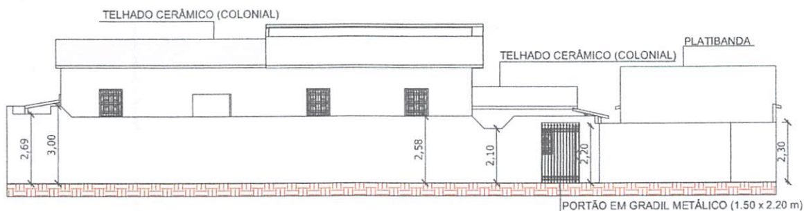
3 FACHADA 1 : 200
