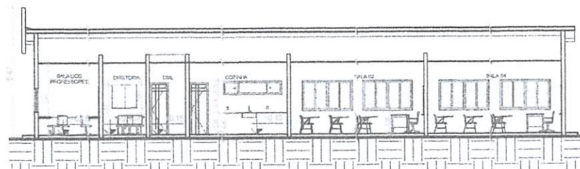
2 Corte 2 1 : 150
