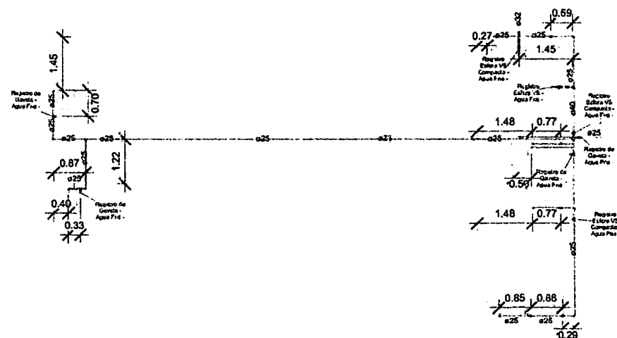
4 ISO-WC PCD
