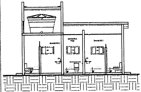
3 Corte 3 1 : 100
