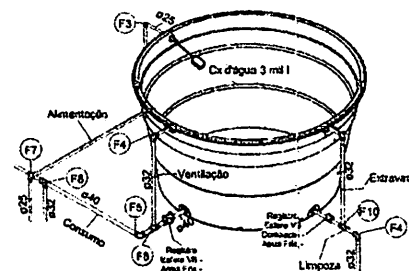
5 ISO-COZ/A.SERVIÇO
