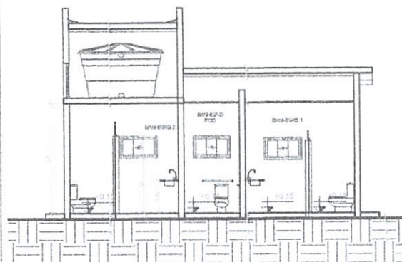
3 Corte 3 1 : 100
