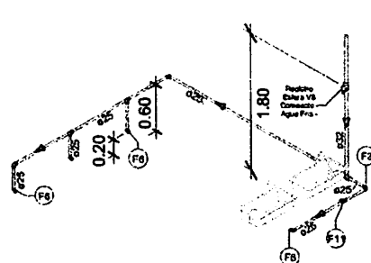
3 ISO-WC FEMININO
