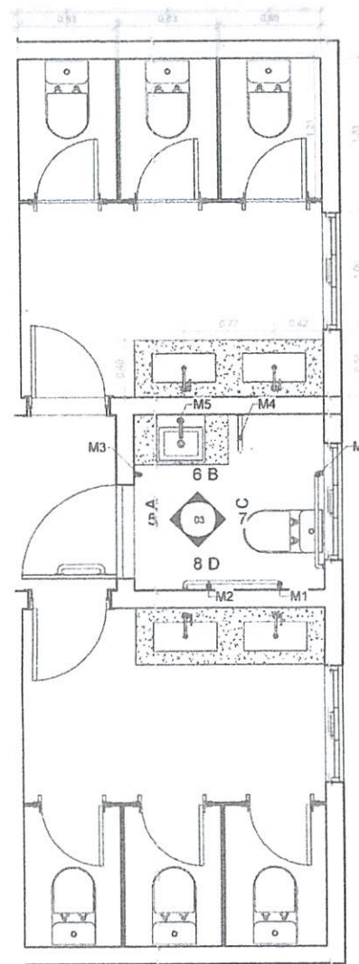
4 DETALHE BANHEIRO 1 : 40
