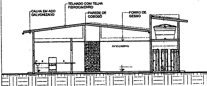
1 Corte 1 1 : 150
