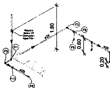
2 ISO-WC MASCULINO
