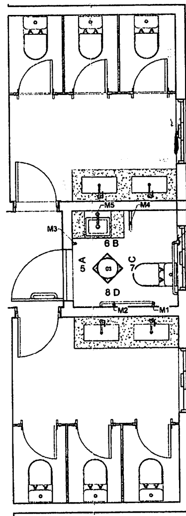
4 DETALHE BANHEIRO 1 : 40
