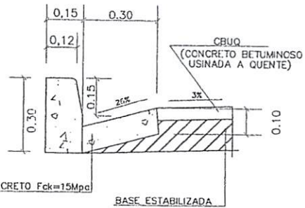
SEÇÃO TRANSVERSAL
