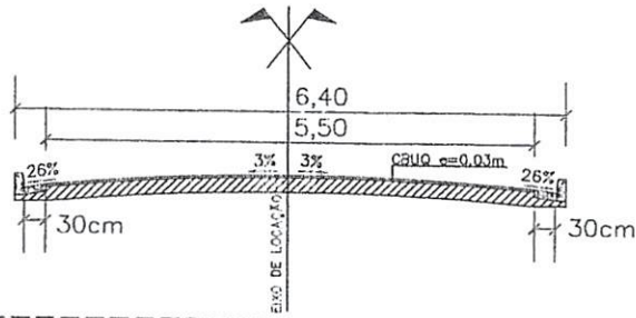
SEÇÃO TRANSVERSAL
