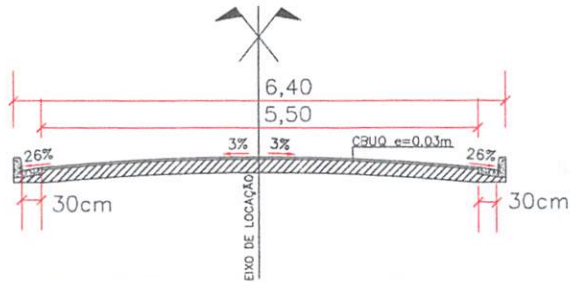
SEÇÃO TRANSVERSAL
