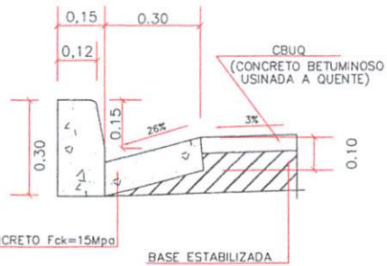
SEÇÃO TRANSVERSAL
