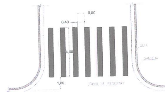
DETALHE DE FAIXA DE PEDESTRE ZEBRADE
