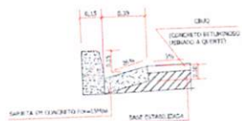
DETALHE: TRECHO SEM CALÇADA
