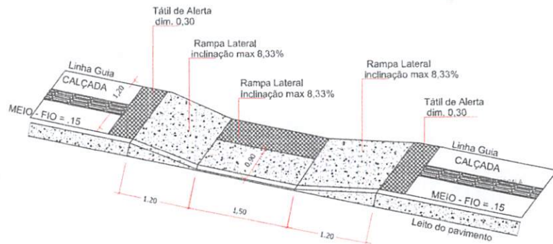
RAMPA - PERSPECTIVA ISOMÉTRICA
