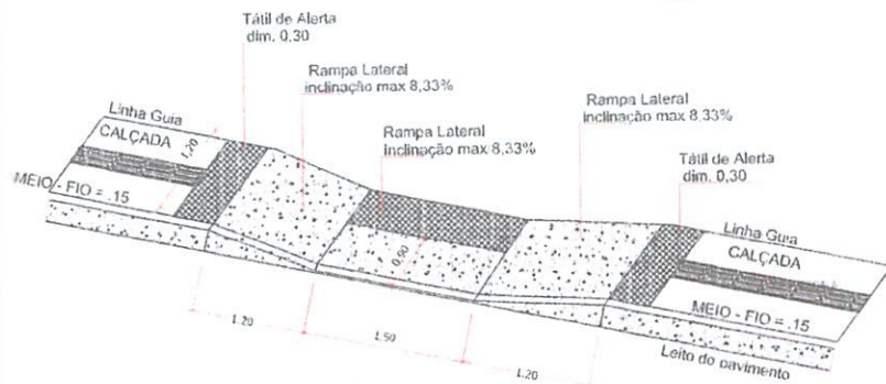
RANPA - RESPECTIVA ISOMETRICA
