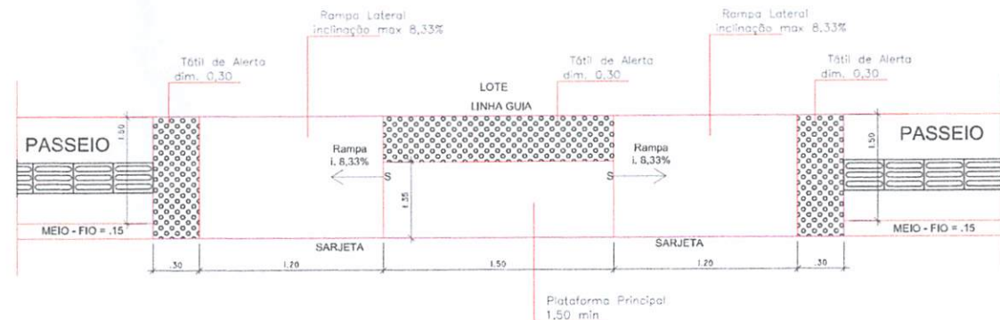
RAMPA - VISTA SUPERIOR
