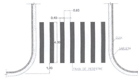
DETALHE DE FAIXA DE PEDESTRE ZEBRADA
