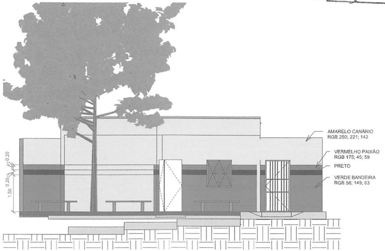
FACHADA FRONTAL 1 : 90
