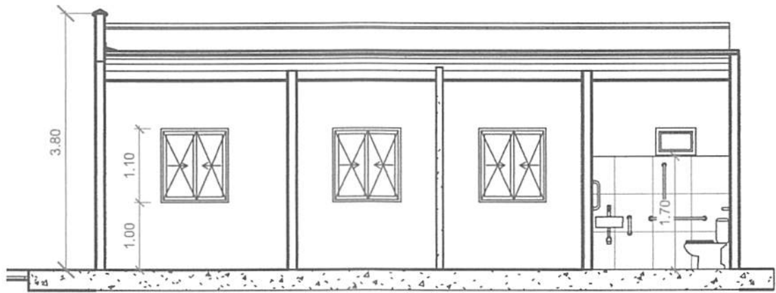
A 1 : 75
