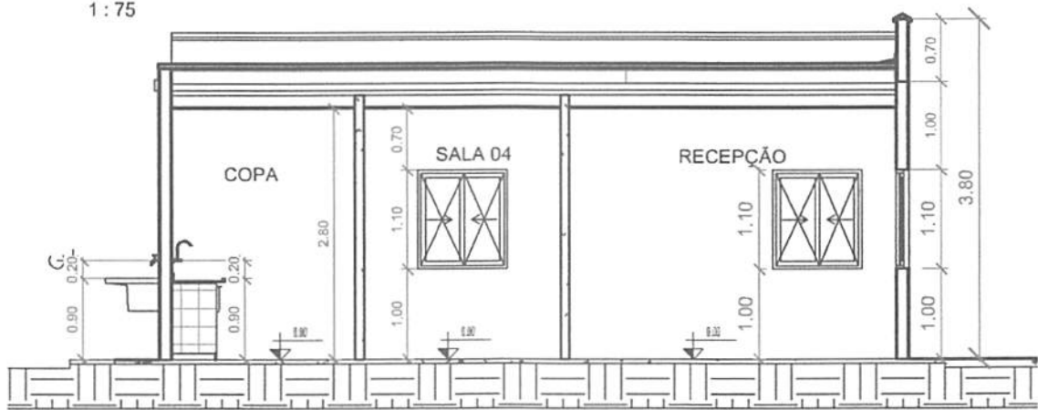
D 1 : 75
