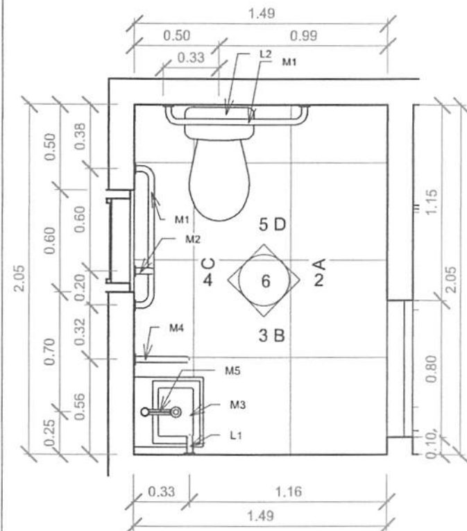
PLANTA BAIXA BANHEIRO 1 : 30
