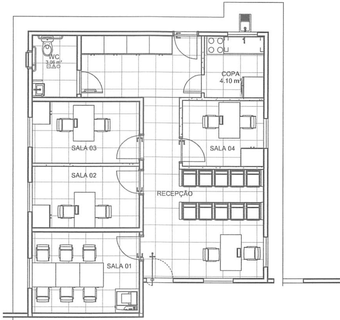
LAYOUT 1 : 75
