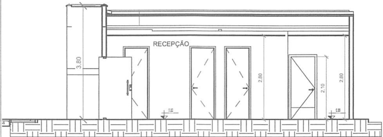
B 1 : 75
