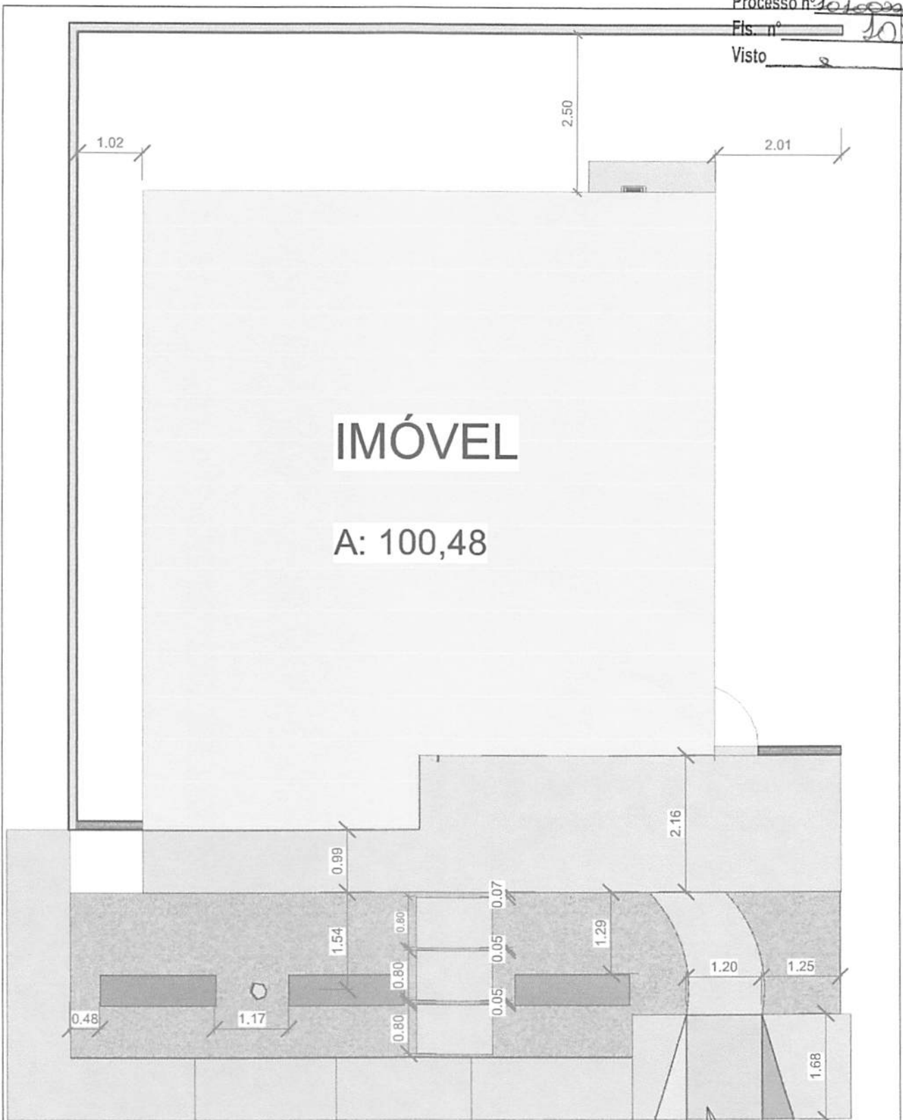
PLANTA DE IMPLANTAÇÃO 1 : 80
