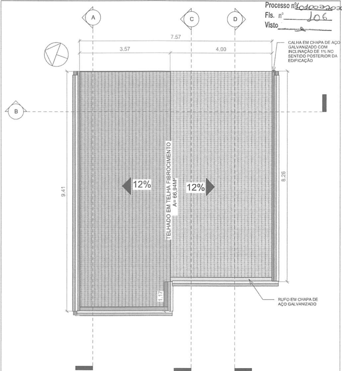
COBERTURA 1:75
