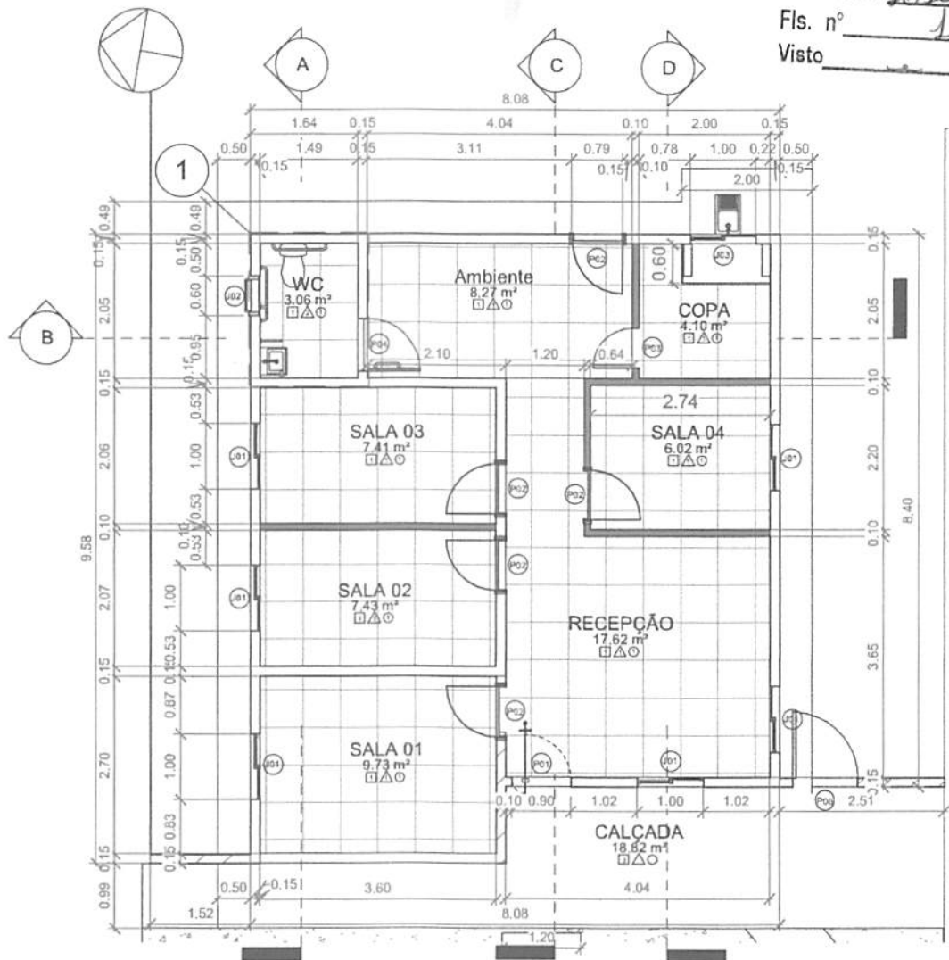
PLANTA BAIXA 1 : 100
