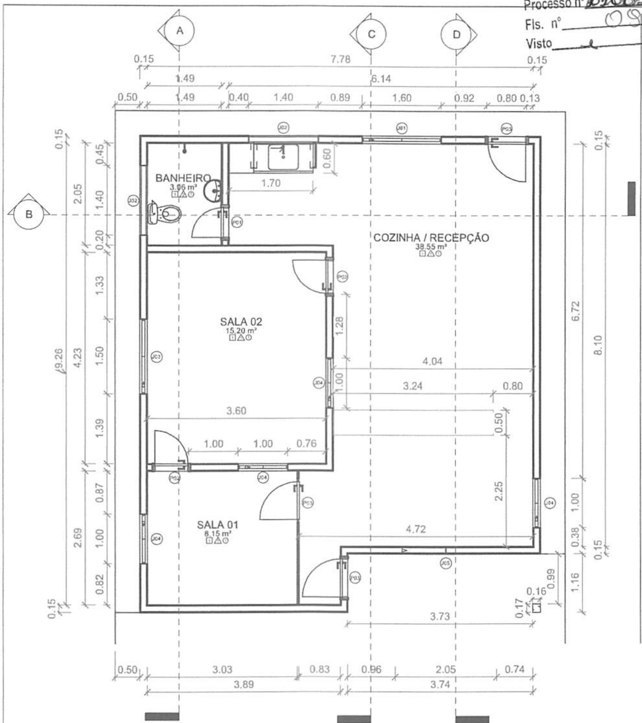
PLANTA BAIXA 1 : 75
