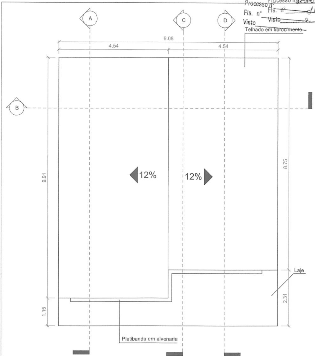
COBERTURA 1 : 75
